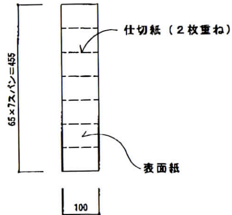
セルバック短辺側面図 1/10
