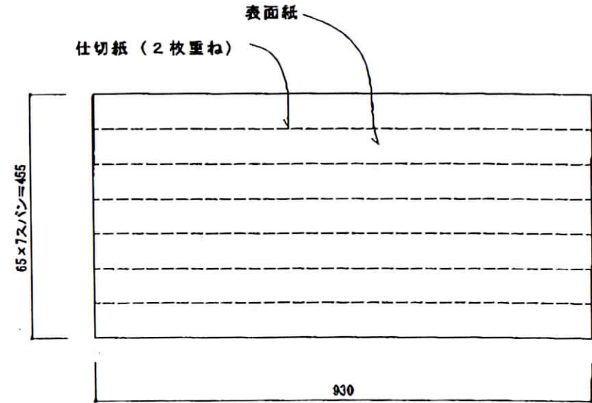
セルバック見下げ図 1/10
